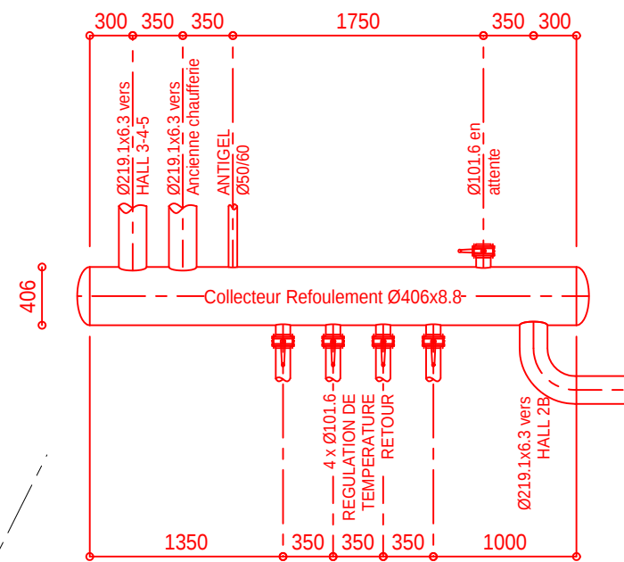
Détail Collecteur Refoulement
