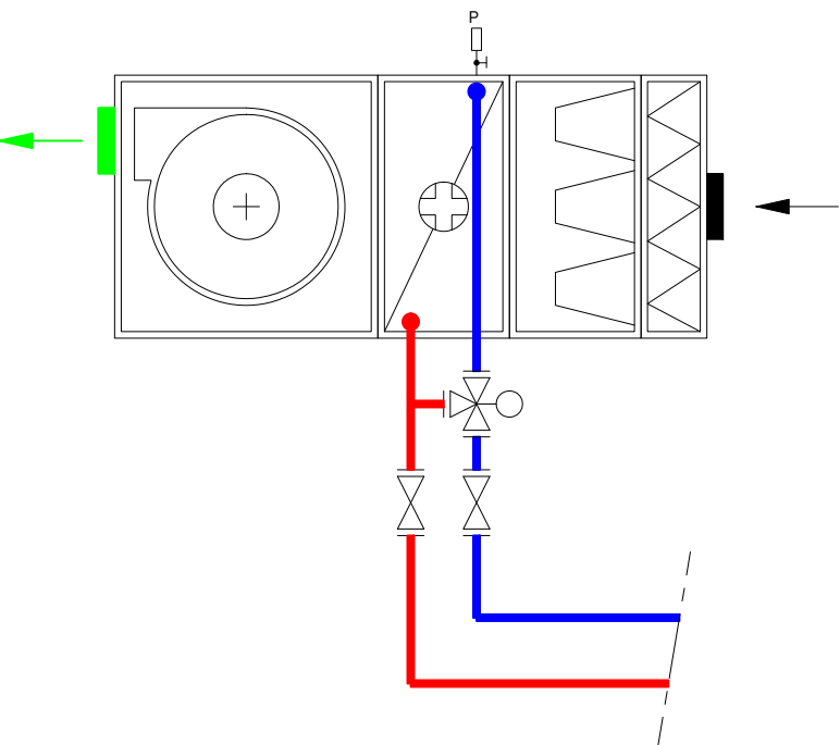
Schéma de Principe C.T.A.
